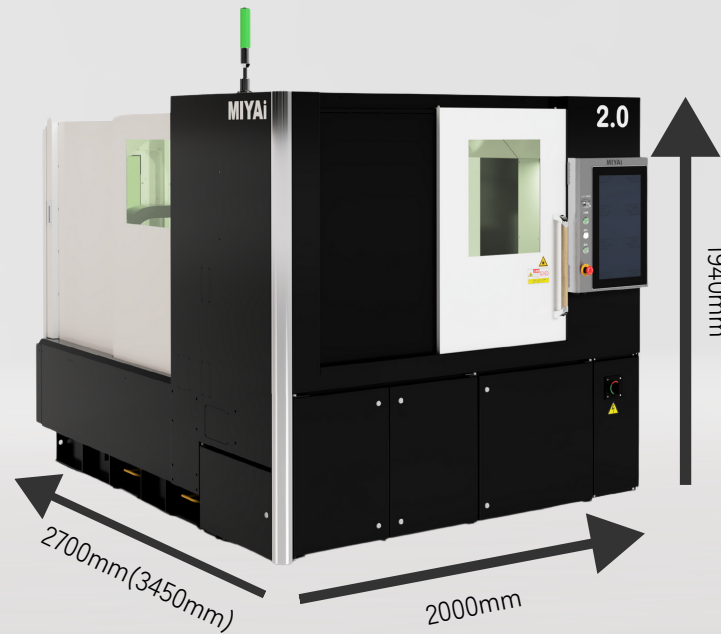
1020×1220mm(1020mm×2020mm)加工機
